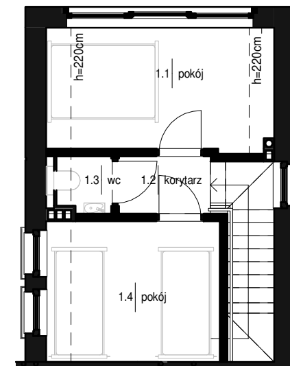
PODDASZE 1:100
