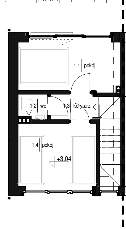
PODDASZE 1:100
