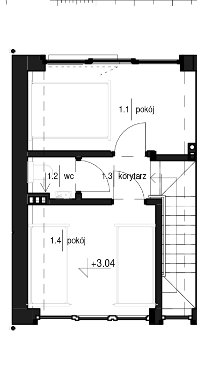
PIĘTRO 1:100
