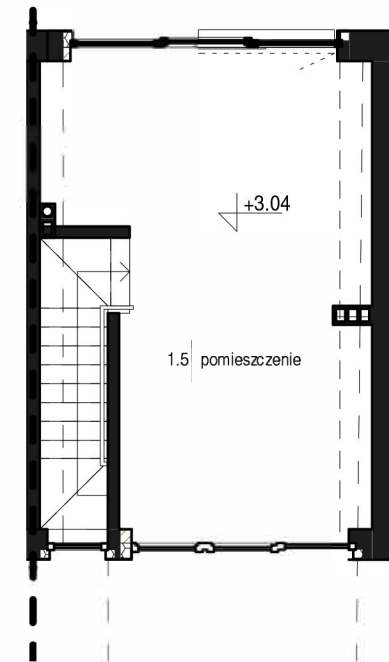
PIĘTRO 1:100
