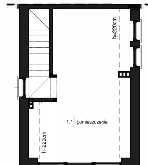
PIĘTRO 1:100
