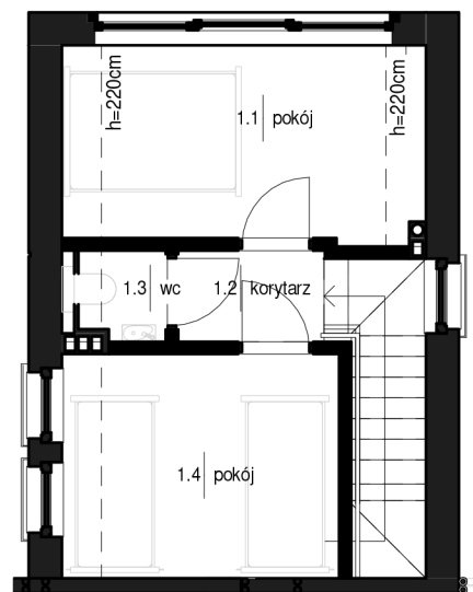
PIĘTRO 1:100
