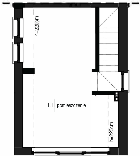
PIĘTRO 1:100
